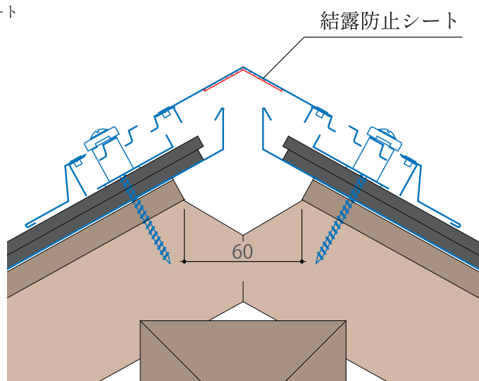
S型換気棟の断面図
