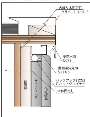
●スレート屋根・化粧破風 施工断面図
