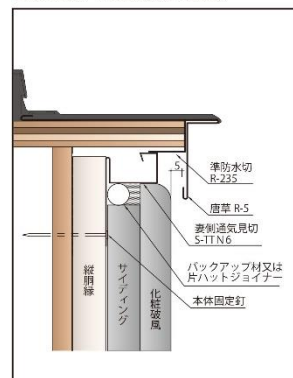
●金属屋根・化粧破風 施工断面図
