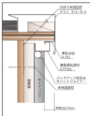
●スレート屋根・サイディング施工断面図
