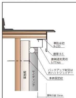
●金属屋根・サイディング施工断面図
