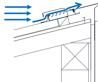
暴風雨時（風圧抜き）
