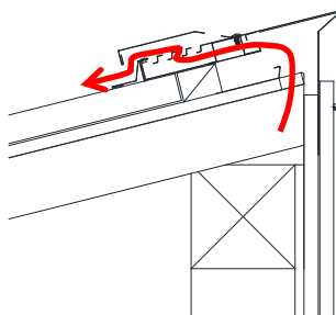
平常時（小屋裏内換気）
