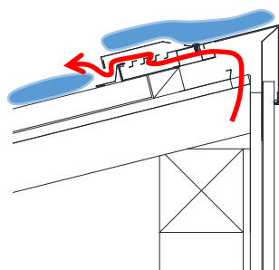
積雪時（小屋裏内換気）
