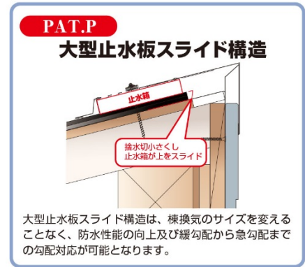
大型止水板スライド構造
